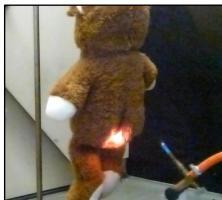
Abbildung 2: Prüfung der Entflammbarkeit
