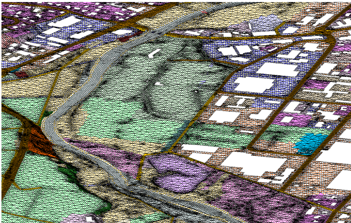
Abbildung 2: Auszug aus dem Berechnungsnetz als 3D-Darstellung mit farblicher Unterscheidung der Rauheitsverteilung, ausgestanzten Gebäuden und variabler Netzauflösung
